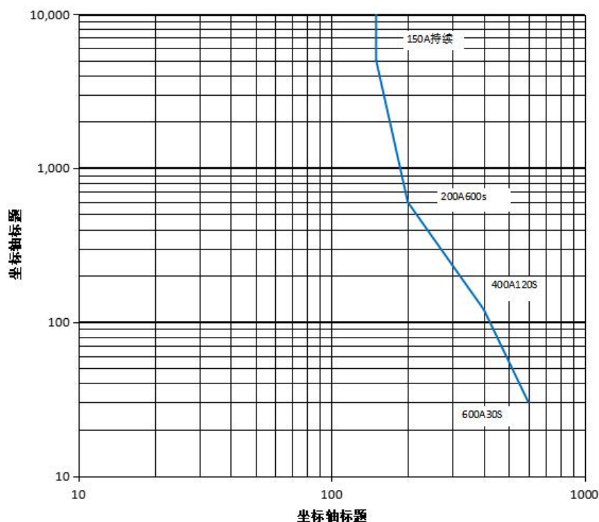
电流耐受曲线
