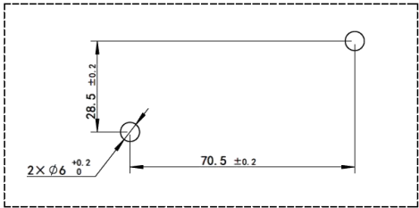
安装孔尺寸
