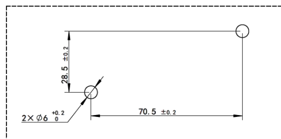
安装孔尺寸
