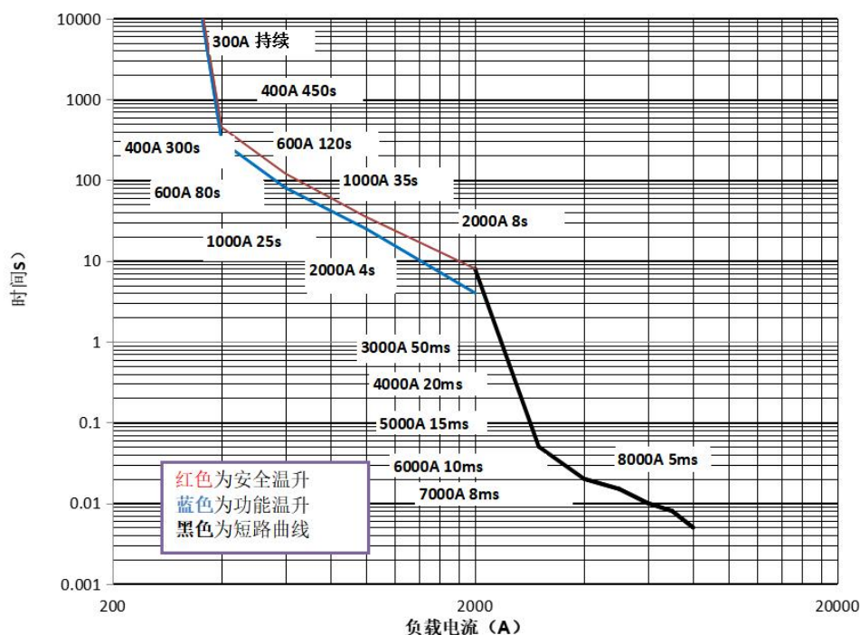
电流耐受曲线
