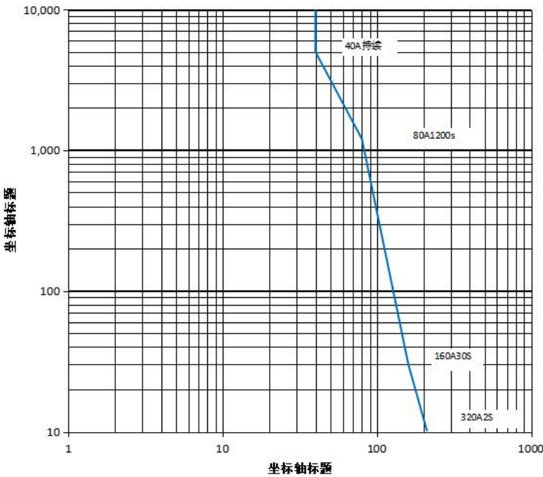
电流耐受曲线
