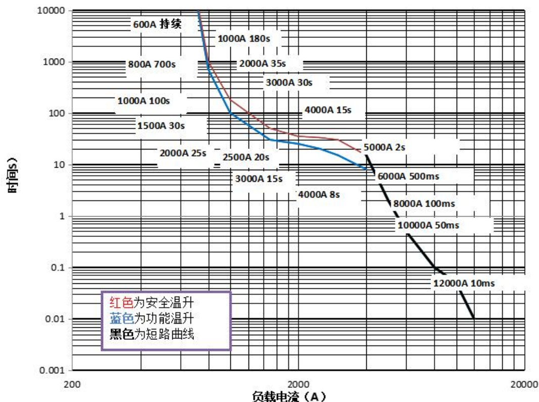
电流耐受曲线
